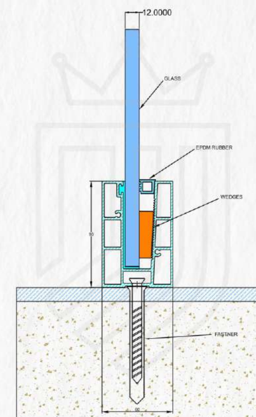
JVL-CP-10 90X60MM
