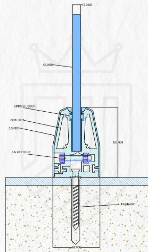
JVL-BKT-01 STEP
